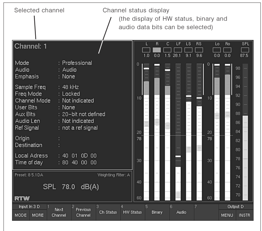
Fig. 1-16: Instrument „AES/EBU-Statusmonitor“ (AES/EBU)
