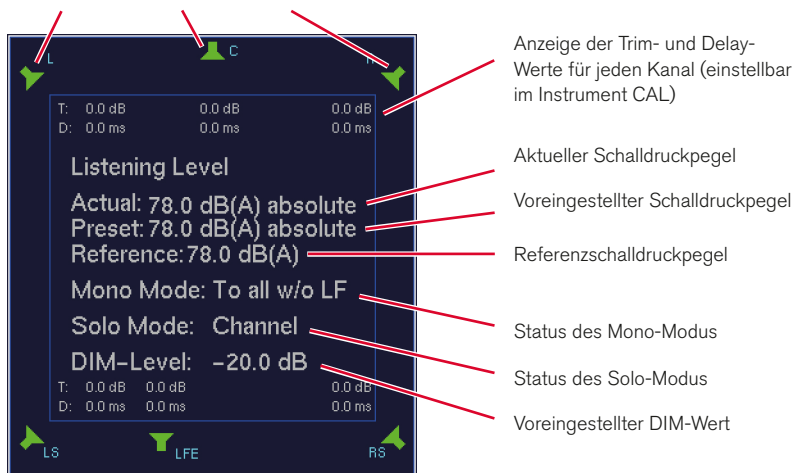
Statusanzeige der zu messenden Kanäle (grün: on, rot: muted)
